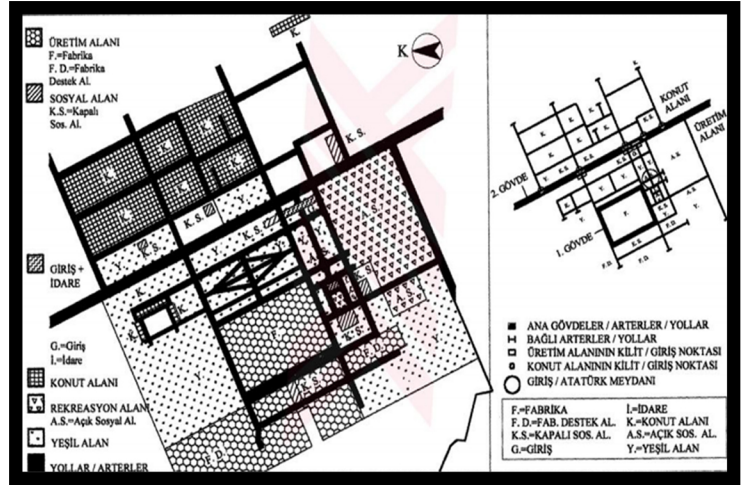
Şekil 4. Sümerbank Yerleşkesi Vaziyet Planı Örneği (Kaynak: Göktaş O. Türkiye’de Lojmanların Oluşumu Ve Bu Oluşumun Temellendirilmesi, 2009)
