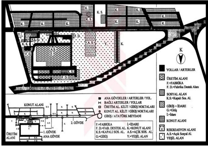
Şekil 3. Sümerbank Yerleşkesi Vaziyet Planı Örneği (Kaynak: Göktaş O. Türkiye’de Lojmanların Oluşumu Ve Bu Oluşumun Temellendirilmesi, 2009)
